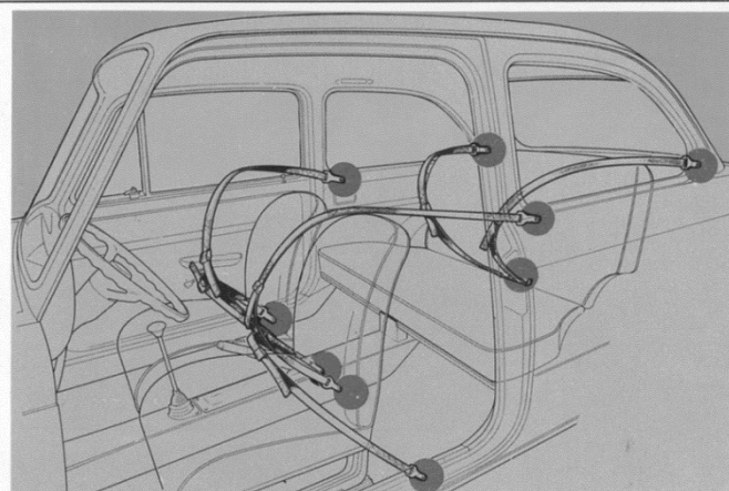
Anschlüsse für die Anbringung von Sicherheitsgurten jeden Typs.
