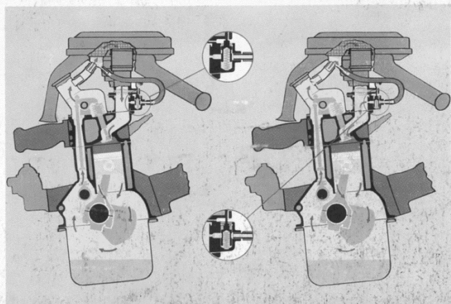
Blow-by-Vorrichtung zum Wiederansaugen der Motorabgase. Ein Beitrag zum Kampf gegen die Verunreinigung der Luft.
